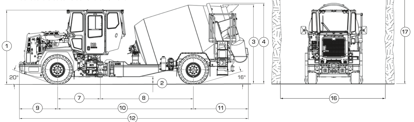
Vue latérale et taille de l'entraînement
